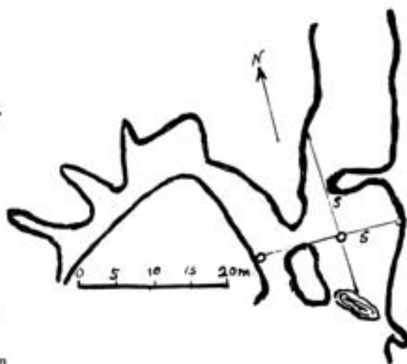
Fig. 2.- Croquis, en planta, de la entrada y vestibulo de Aitzbitarte IV.
