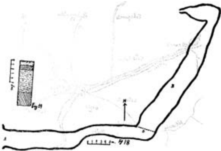
Figs. 18 y 19. — 18: Croquis, en planta, de la cueva de Atabo (de un apunte de 1920). A D, la parte destruida; B, la parte que en 1957 se conservaba todavía. — 19: Corte del yacimiento en su portal.
