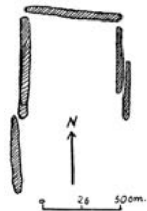
Fig. 11. — Dolmen de Aitxu; cámara incompleta en medio de un túmulo de piedras esquinadas cuya base tiene un diámetro de 8 metros y cuya altura mide tan sólo 0,80 m.
