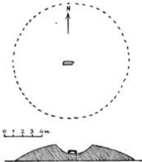
Fig. 1. — Dolmen de Petilarre; croquis en planta y corte.
