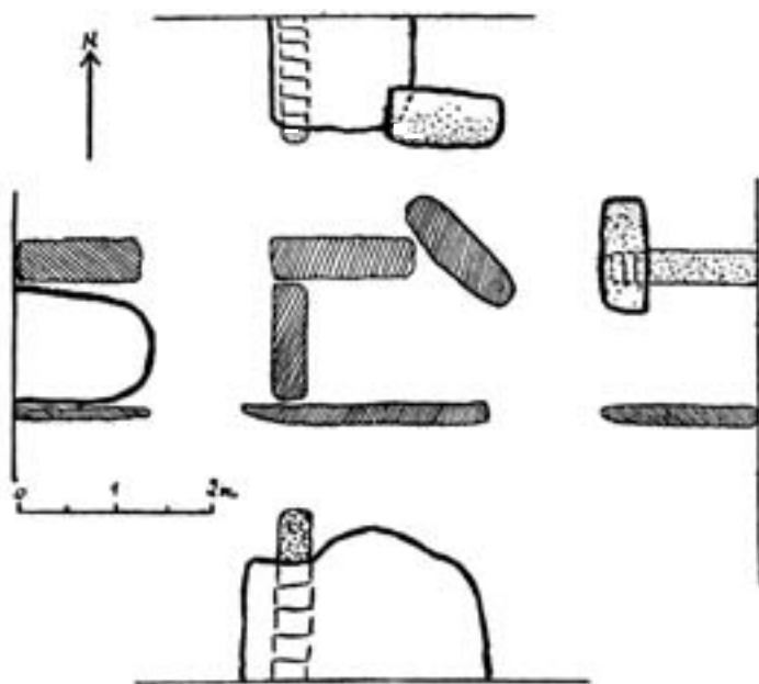
Fig. 3. — Dolmen de Arrondo.
