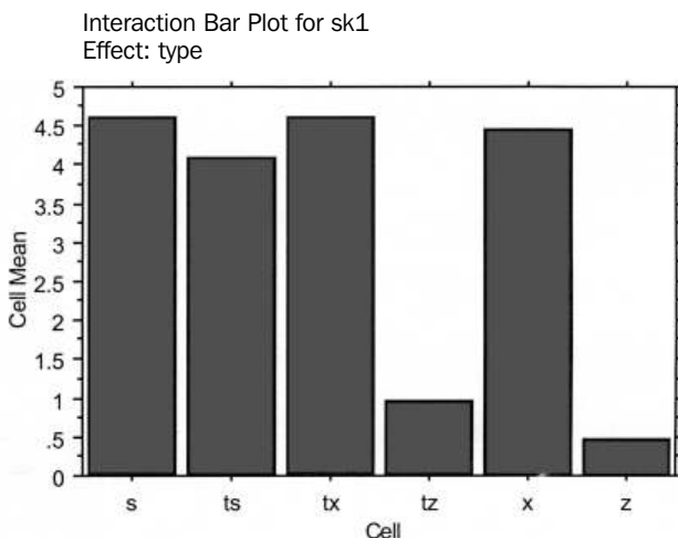
Fig. 5. Skewness
